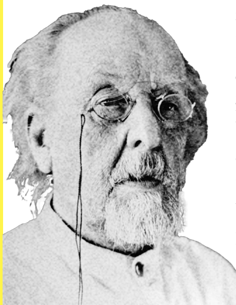
Konstantin Tsiolkovsky
